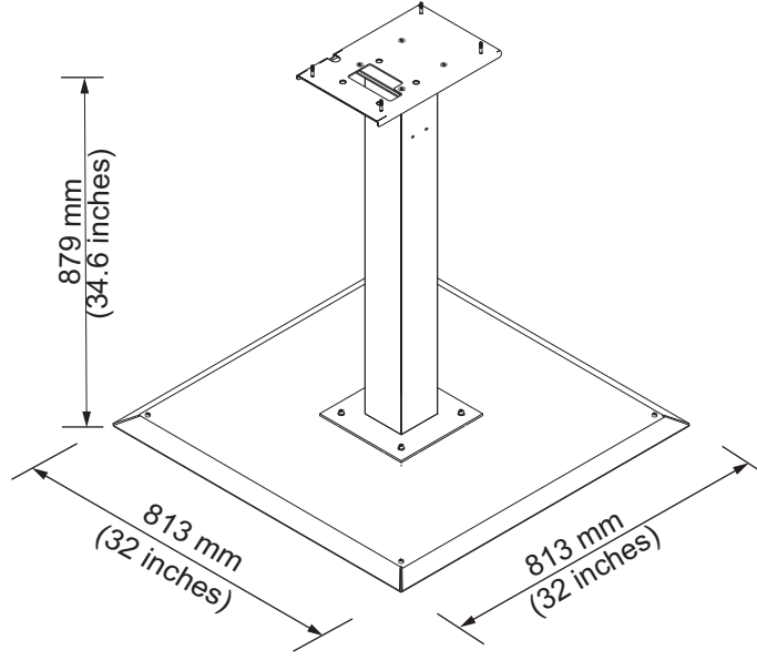
Şekil A-4: Sabit Yazıcı Standı
