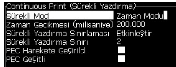
Şekil 4-28: Zaman Modu
