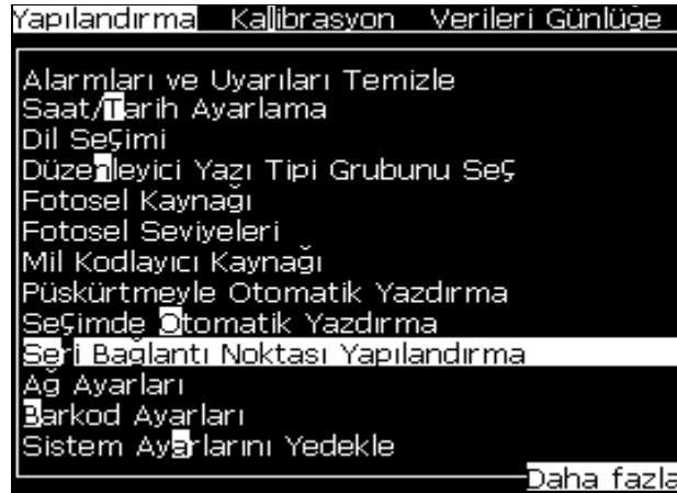
Şekil 4-20: Yapılandırma Menüsü
