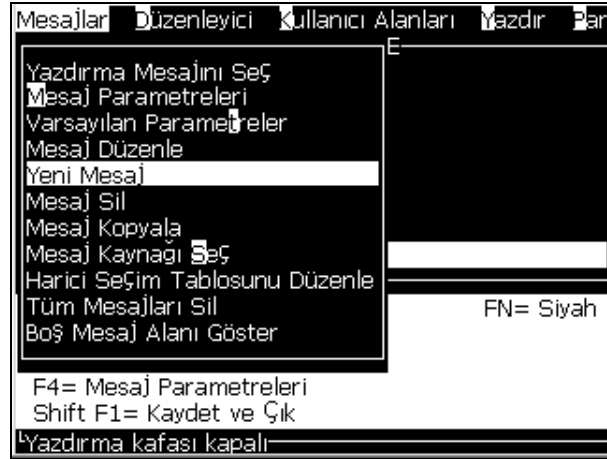
Şekil 5-3: Mesajlar Menüsü
