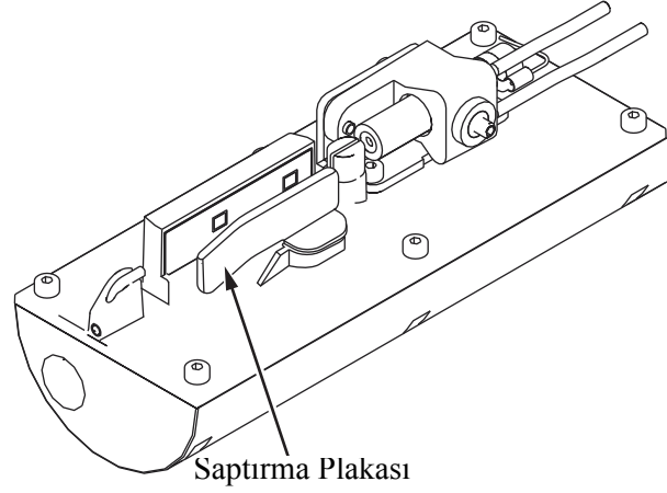
Şekil 6-5: Saptırma Plakasını Temizleme
