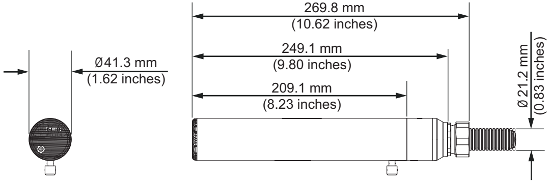
Yazıcı Kafası
