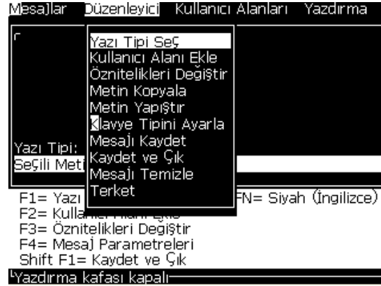
Şekil 5-48: Düzenleyici Menüsü
