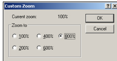
Şekil 5-58: Özel Yakınlaştırma
