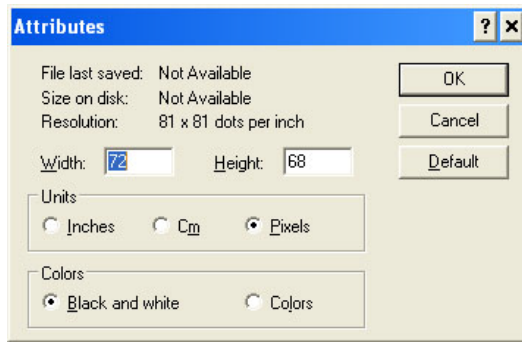
Şekil 5-59: Görüntü Öznitelikleri
